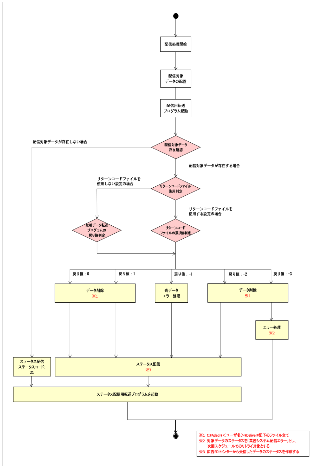
図 2-3 転送プログラム起動後処理フロー(受信時)
