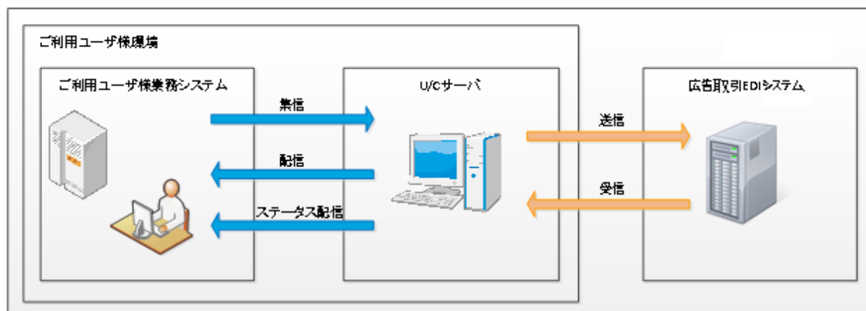
図 1-1 広告取引EDIシステム⇄U/Cサーバ⇄業務システム 関係図
