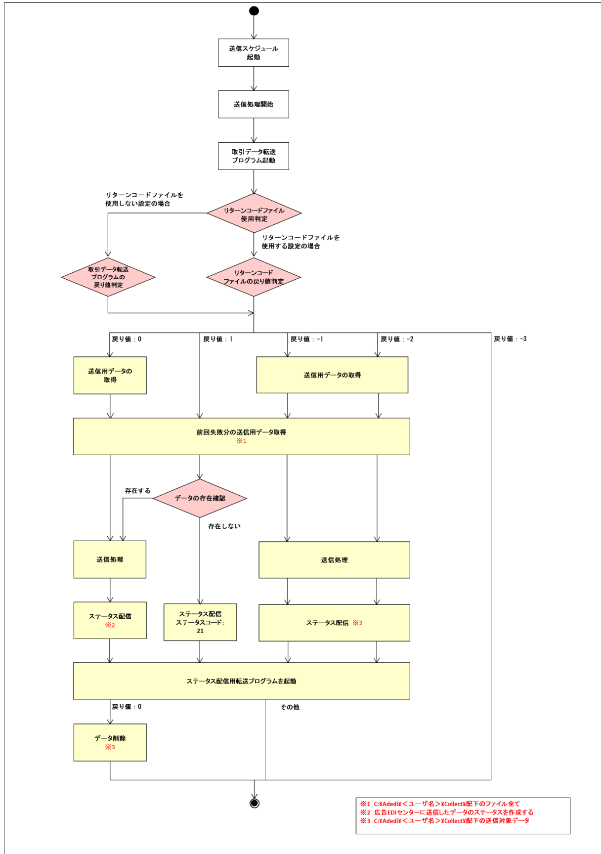
図 2-2 転送プログラム起動後処理フロー(送信時)
