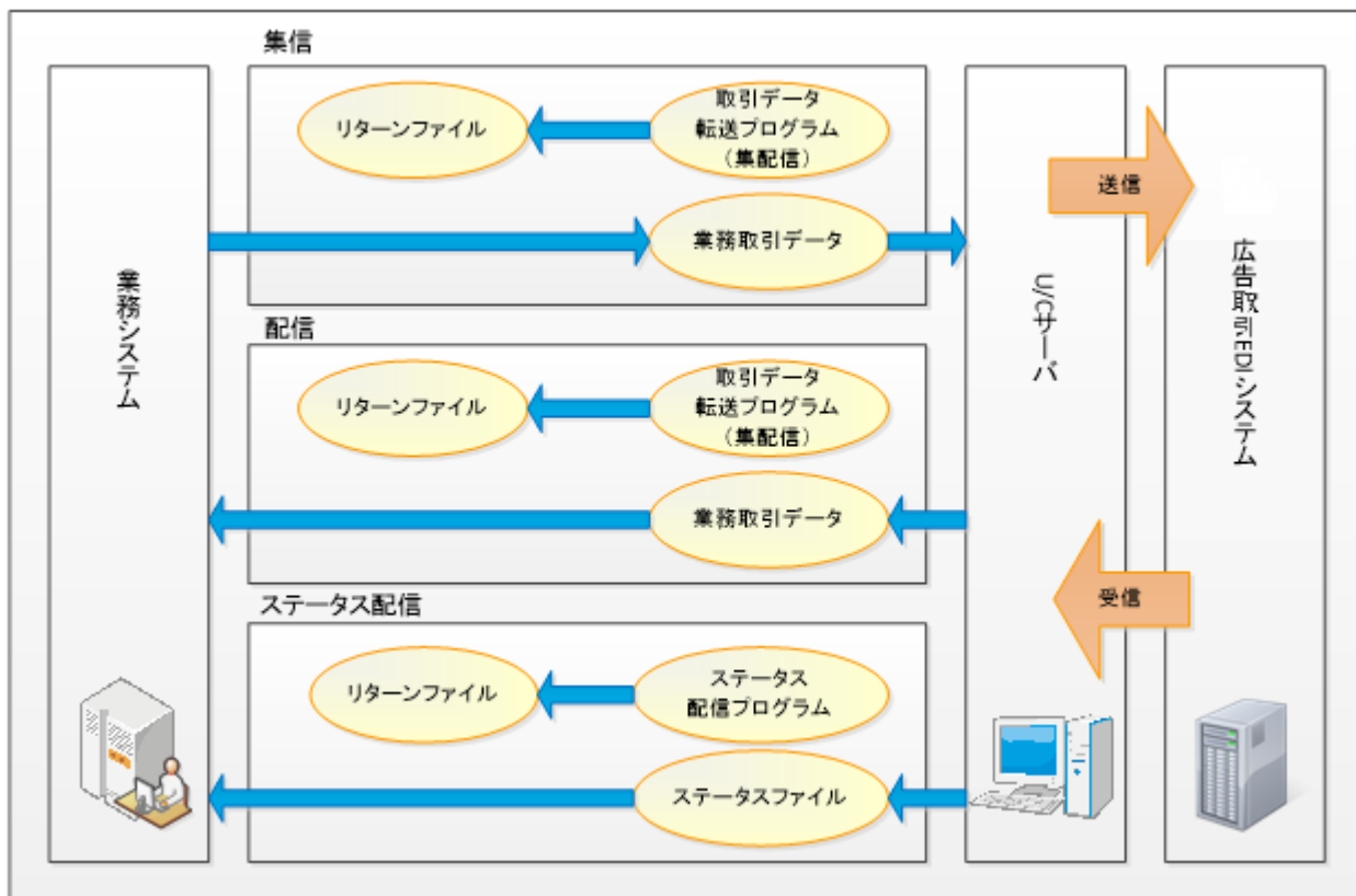
図 2-1 U/Cサーバ-業務システム インターフェースイメージ図
